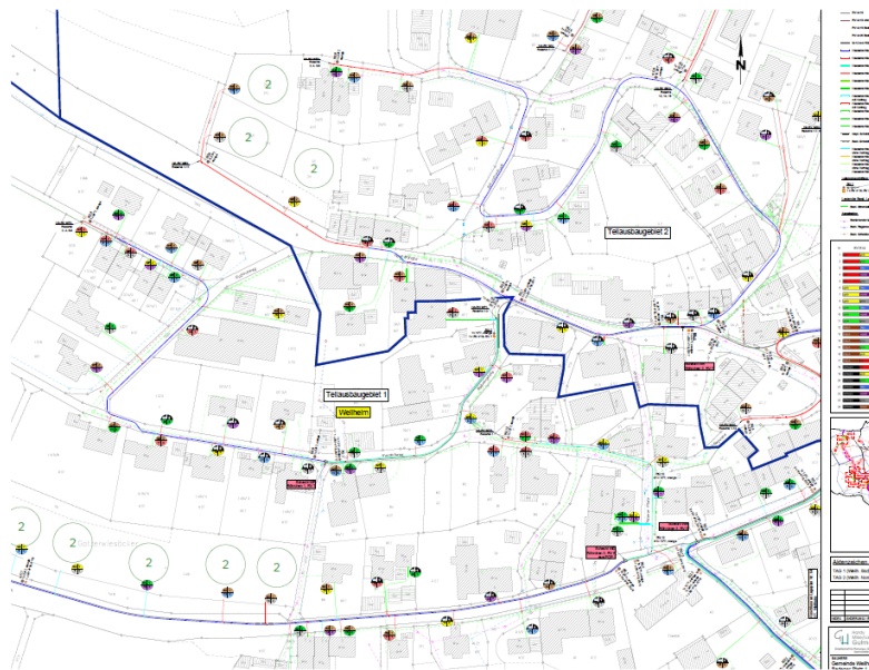
Detailauszug Ortsteil Weilheim / Ausführungsplanung
